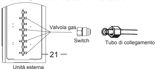
Unità esterna
